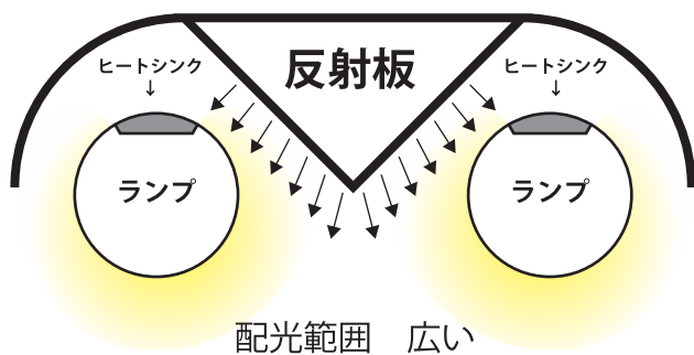
弊社製品：Le:dim- S32W Type 型番：SFL1198-T8-K52-36V 外形寸法：管径 25.5mm 管長 1,198mm 照射角度：300℃
